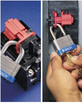
Şalter Tutucu Bileşenler - Engelleme Çubuğu Tutucu
