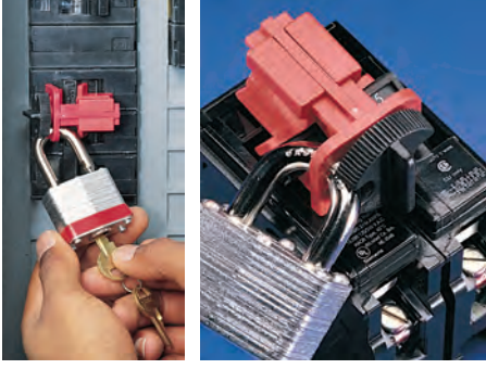
Üniversal multipole şalter kilidi, aralarında bar olan ikili veya üçlü şalterleri kilitlet.
