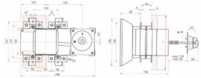
T1-T1 Size (6 pole 250A-315A)
