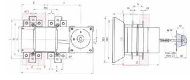
T2-T2 Size (6 pole 630A)
